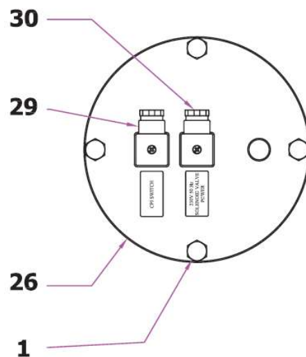
Вид сверху на крышку (26)
